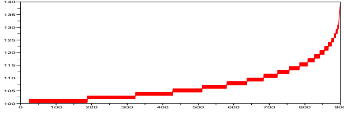
FIG. 1 – Tracé de la frontière d'exercice du put américain à la monnaie dans un modèle de Cox, Ross et Rubinstein avec \sigma = 0.4 , r = 0.05 , T = 1 , et n = 900 .
