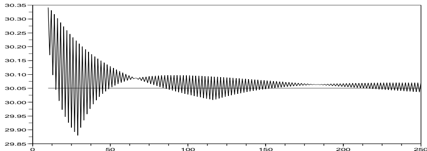
FIG. 1 – Tracé du prix Cox, Ross et Rubinstein C_0(n) d'un Call Européen en fonction de n et de sa limite, le prix Black-Scholes. Valeur des paramètres : S_0 = 140 , \sigma = 0.40 , r = 0.05 , et K = 130
